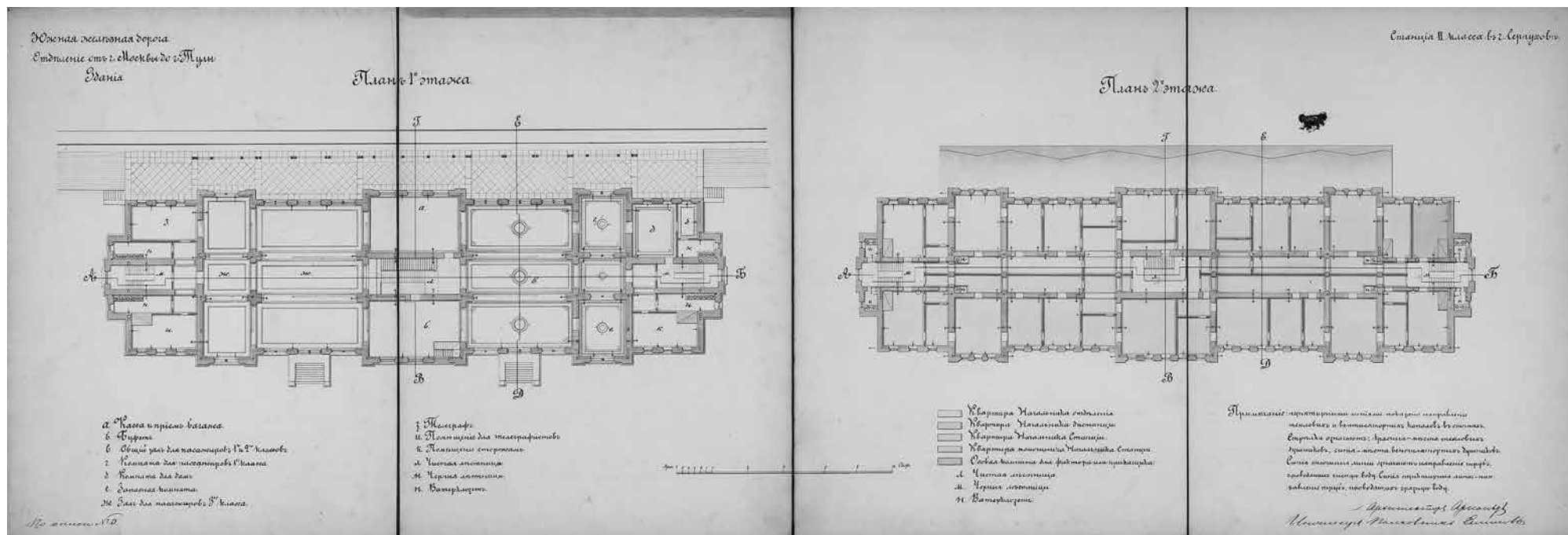
1. Максимилиан Арнольд. Проект пассажирского здания на станции II класса в Серпухове. Планы 1-го и 2-го этажей РГИА. Ф. 350. Оп. 29. Д. 104. Л. 1
