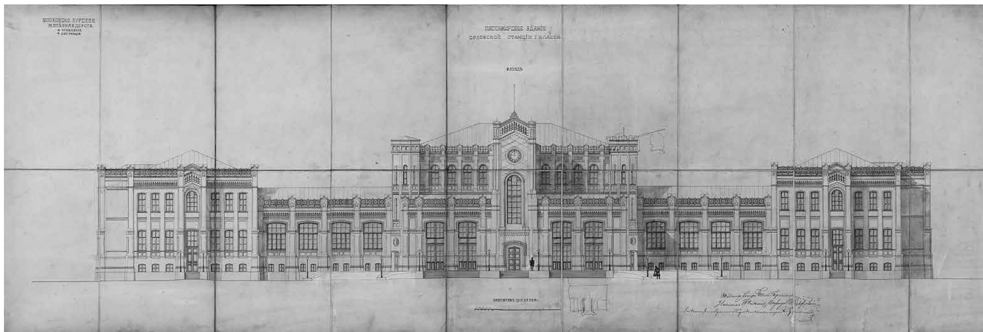
9. Иосиф Тибо-Бриньоль. Проект пассажирского здания на станции I класса в Орле. Фасад РГИА. Ф. 350. Оп. 29. Д. 103. Л. 96–100
