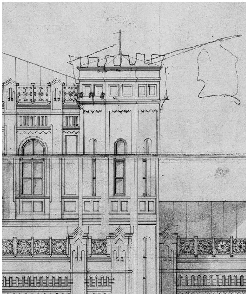
10. Иосиф Тибо-Бриньоль. Проект пассажирского здания на станции I класса в Орле. Фасад. Фрагмент РГИА. Ф. 350. Оп. 29. Д. 103. Л. 96–100
