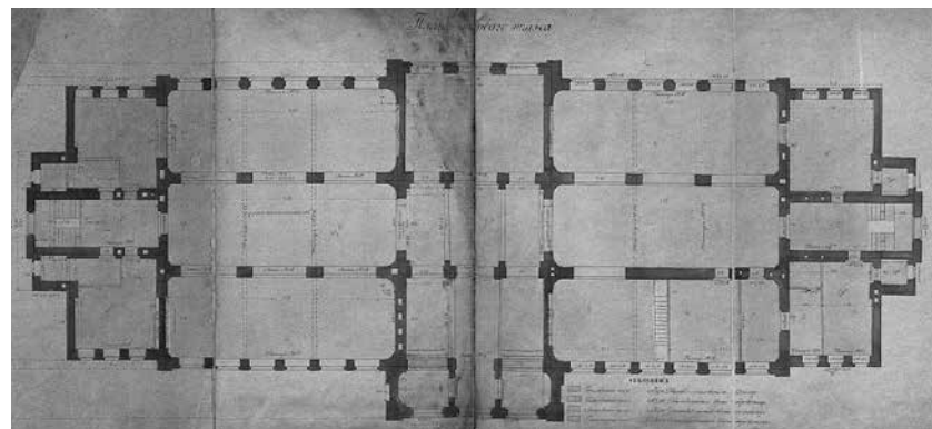
2. Исполнительный чертеж пассажирского здания на станции II класса в Серпухове. План 1-го этажа ЦГАМ. Ф. 413. Оп. 25. Д. 151. Л. 10
