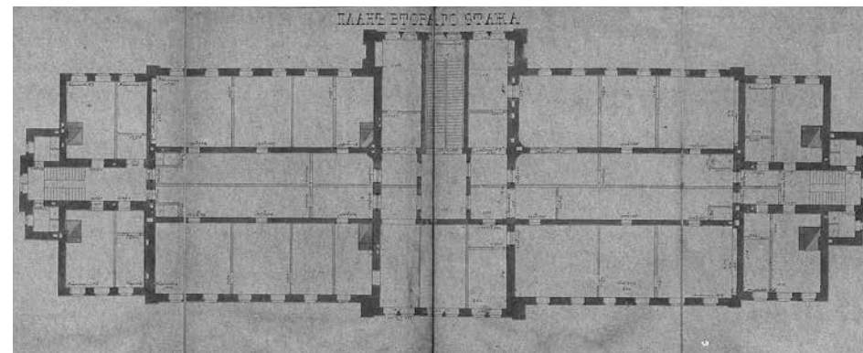
3. Исполнительный чертеж пассажирского здания на станции II класса в Серпухове. План 2-го этажа ЦГАМ. Ф. 413. Оп. 25. Д. 151. Л. 11
