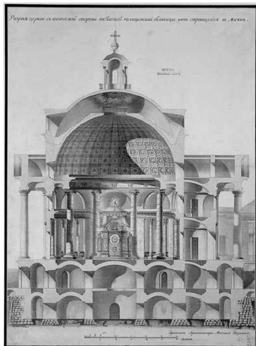
4. Матвей Казаков. Москва. Голицынская больница. Разрез церкви с восточной стороны. 1790-е 5-й альбом Казенных строений ГНИМА, РІ-12291/34
