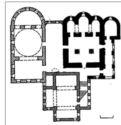
2. Собор Вознесения Господня Вознесенской Давидовой пустыни План [13, с. 314]
